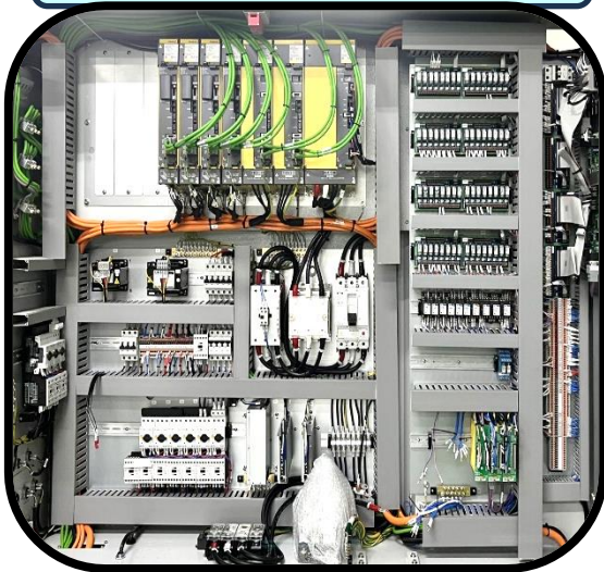
M/c Retrofitting
